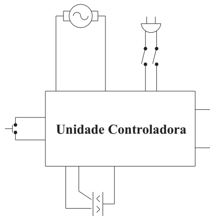
Diagrama de Ligação Mod. ABN
