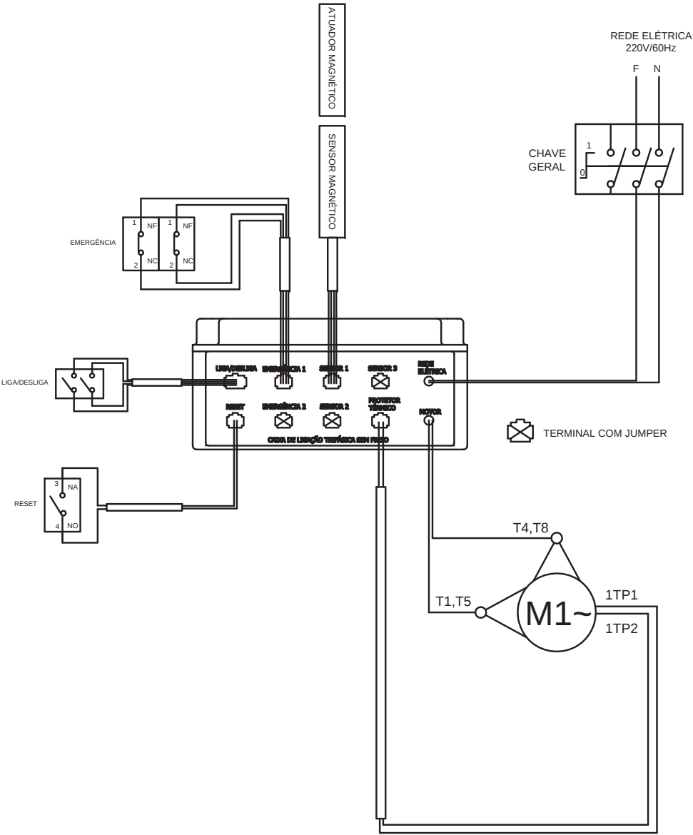
Código do Diagrama Elétrico: 47886.5 Versão do Diagrama Elétrico: Versão 01
