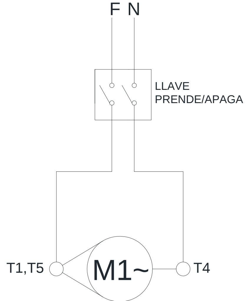
Diagrama Eléctrico: 49841.6
