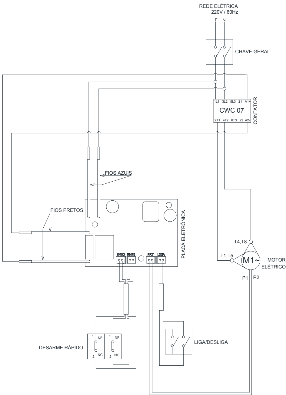
Código do Diagrama Elétrico: 53240.1
