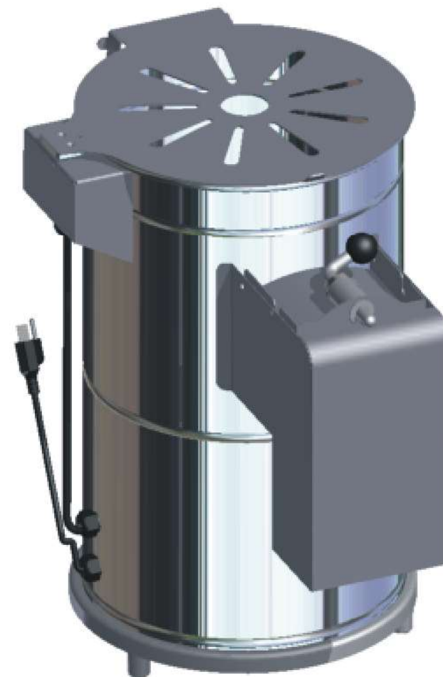
PELADORA DE PAPAS, INOXIDABLE, 6 kg
